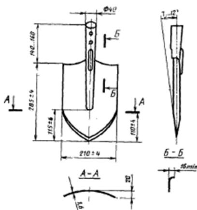
Рисунок 1.1 — Лопата копальная остроконечная, ЛКО
