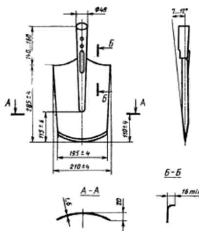
Рисунок 2 — Лопата копальная прямоугольная, ЛКП Примечание. Источник: [1, С. 5]
